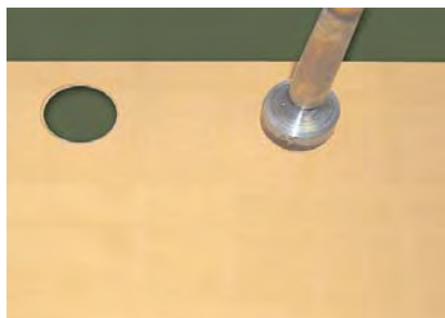
прожечь отверстия (z.B. номер артикула 31 052 + 31 053) с помощью нагретого резака*/ melt out marked holes with hot cutter (e.g. art. no. 31 052 + 31 053)
