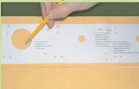
Schablone (z.B. Art. Nr. 31035) ausbrechen, aufstecken und Löcher markieren/ break out hole model (e.g. art. no. 31035), pin it and mark the holes
